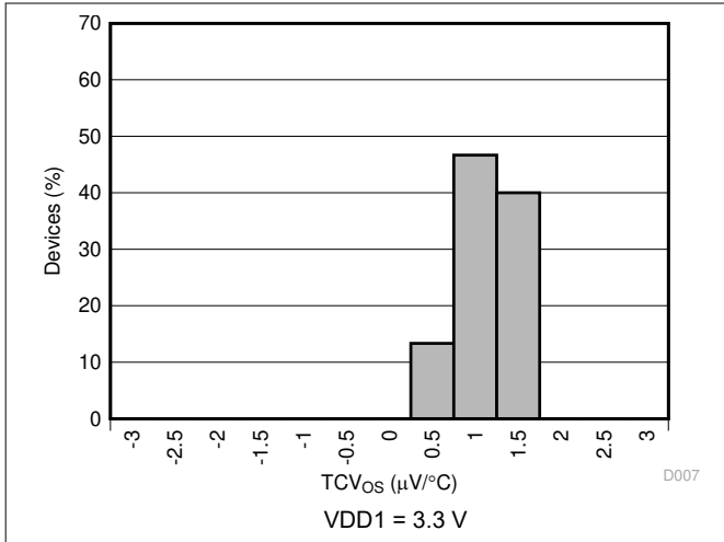
图 6-11. Input Offset Drift Histogram
