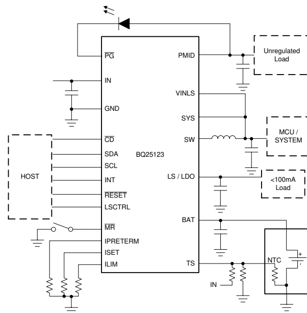
简化原理图
