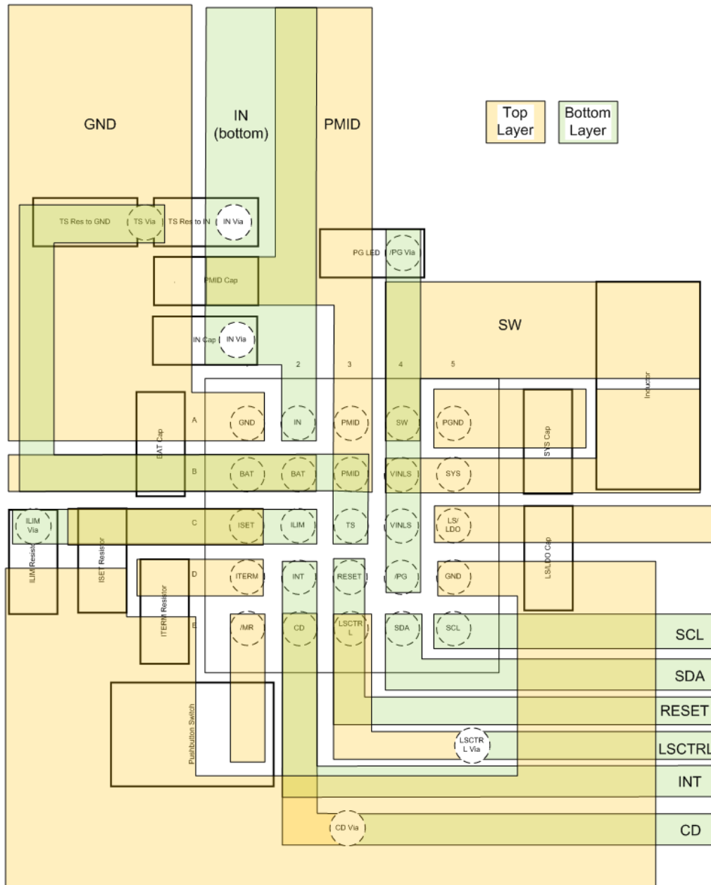
图 11-1. BQ25123 Layout
