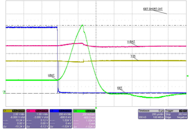
图 8-9. ISET Short-Circuit Response
