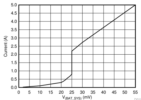
图 8-4. BATFET V-I Curve
