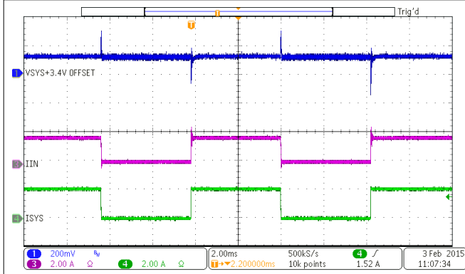
图 9-4. Charge Enable
