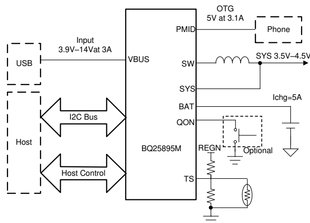
简化原理图
