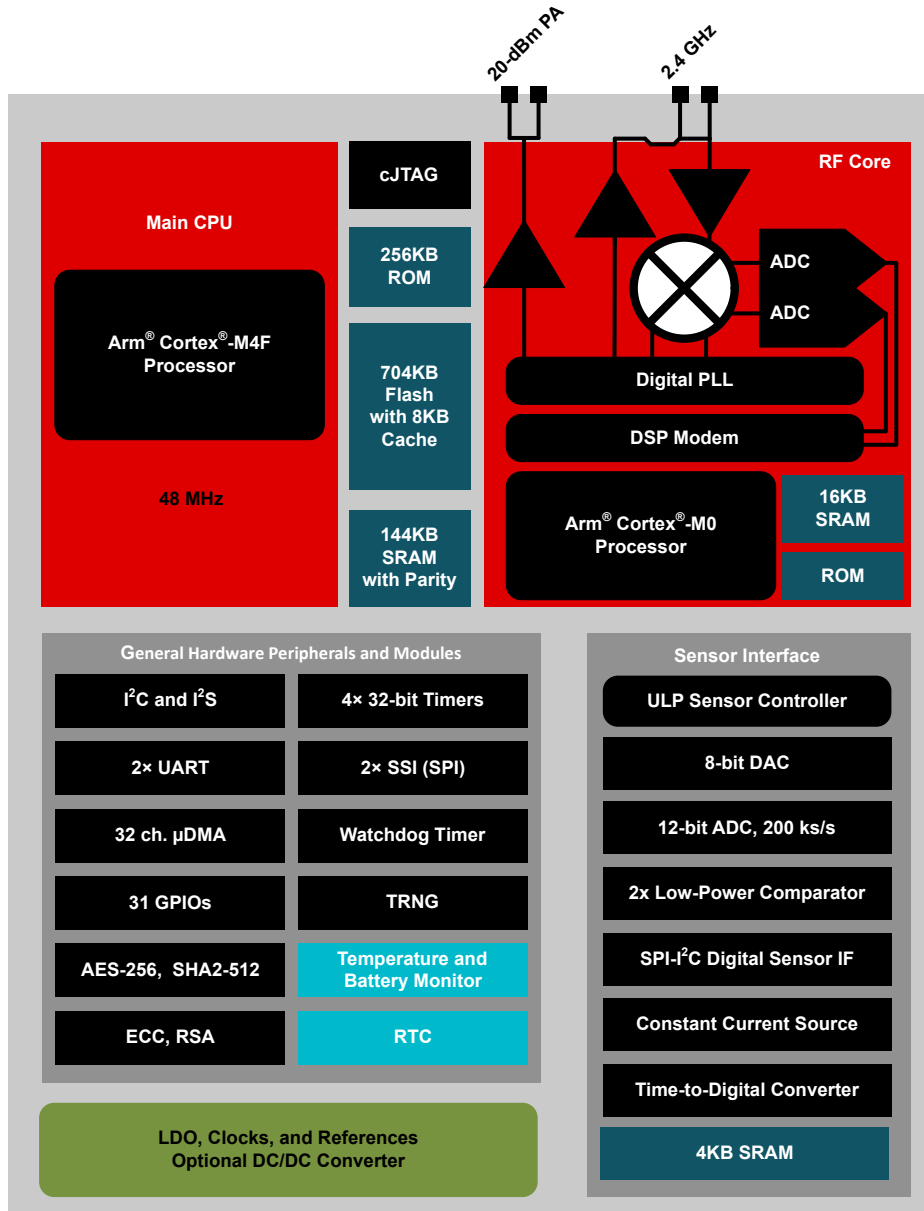
图 3-1. CC2652P7 方框图
