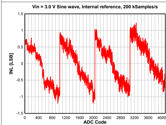
图 8-23. INL versus ADC Code
