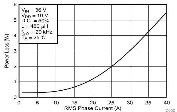
功率损耗与输出电流
