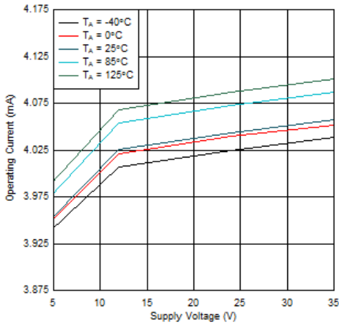
图 6-4. 工作电流与电源电压之间的关系
