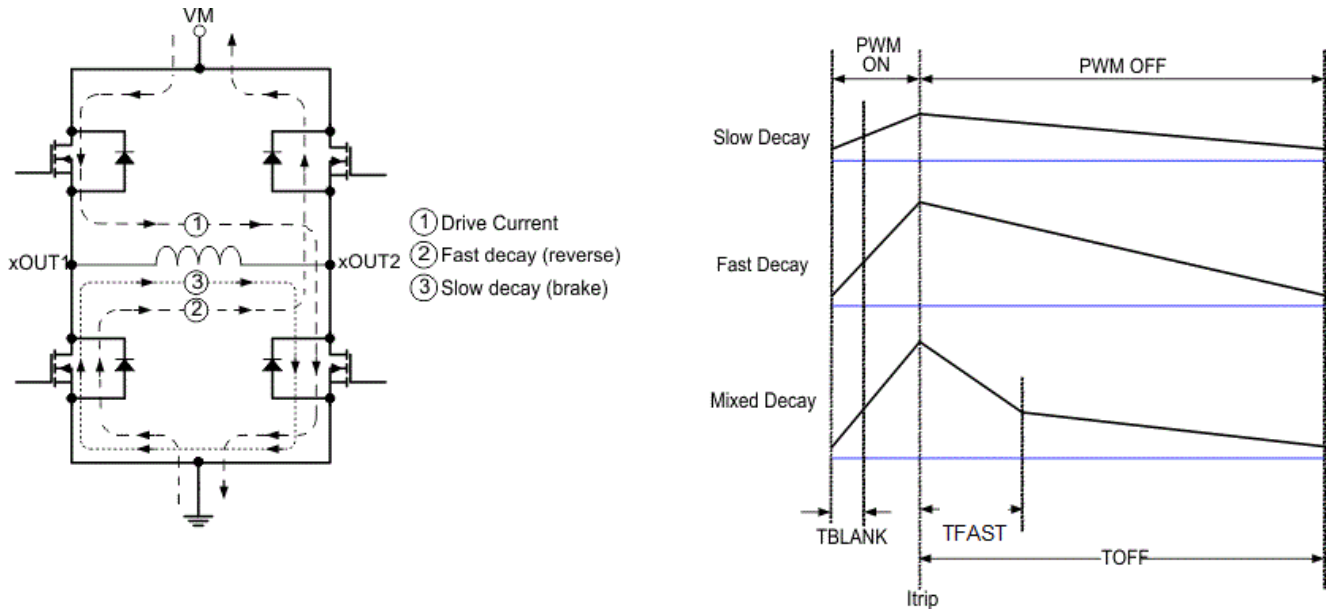
图 7-7. 衰减模式
