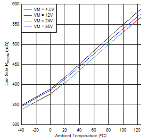
图 6-7. 低侧 R_{DS(ON)} 与温度间的关系
