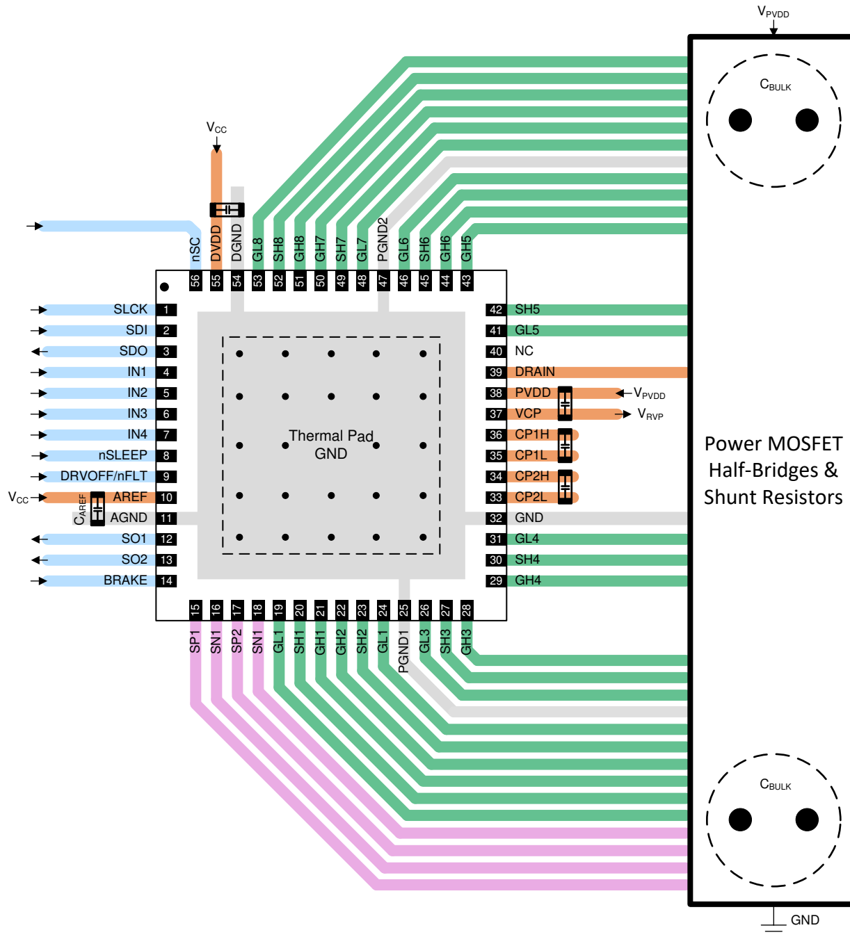
图 11-1. Layout Example
