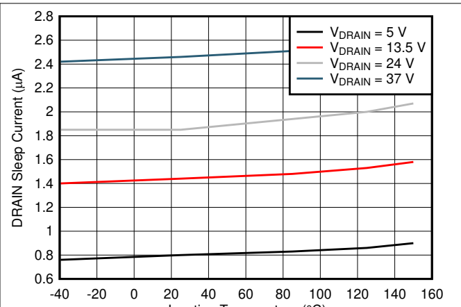
图 7-3. DRAIN Sleep Current
