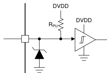
图 8-23. Input Pin Structure (nSCS)
