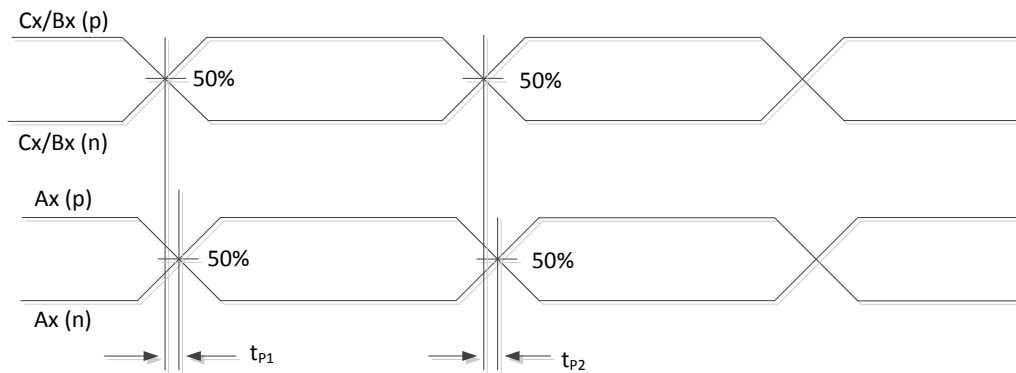
Inter-pair skew
