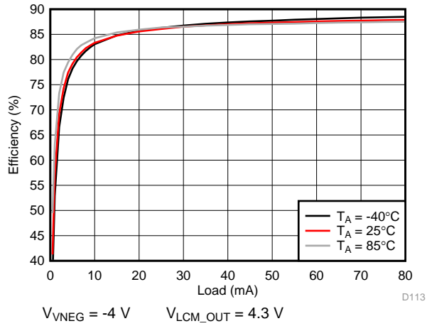
图 199. VNEG Efficiency
