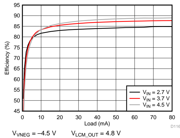
图 202. VNEG Efficiency
