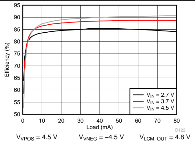
图 208. VPOS/VNEG Efficiency
