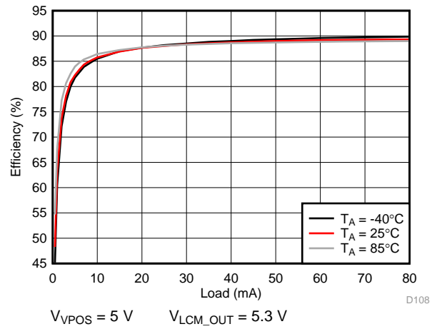
图 194. VPOS Efficiency
