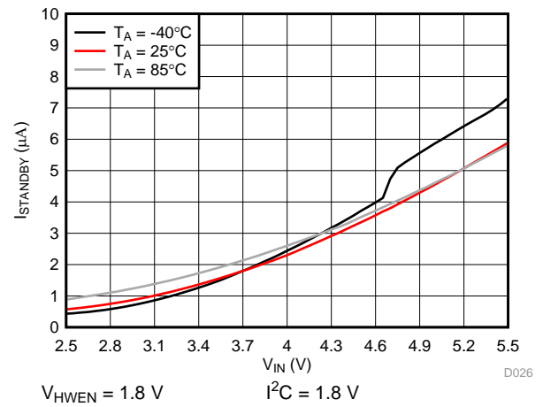
图 29. I_q Standby
