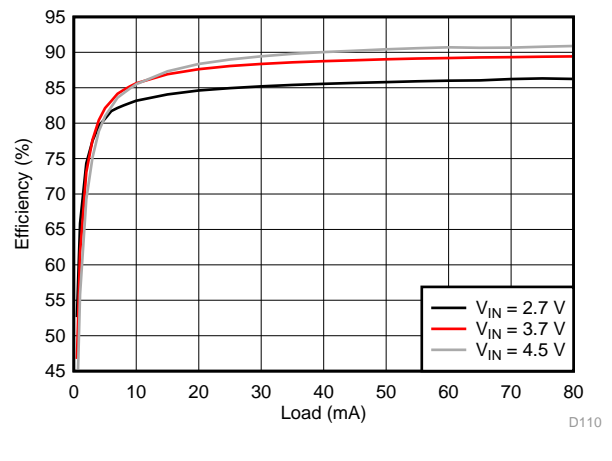
图 196. VPOS Efficiency
