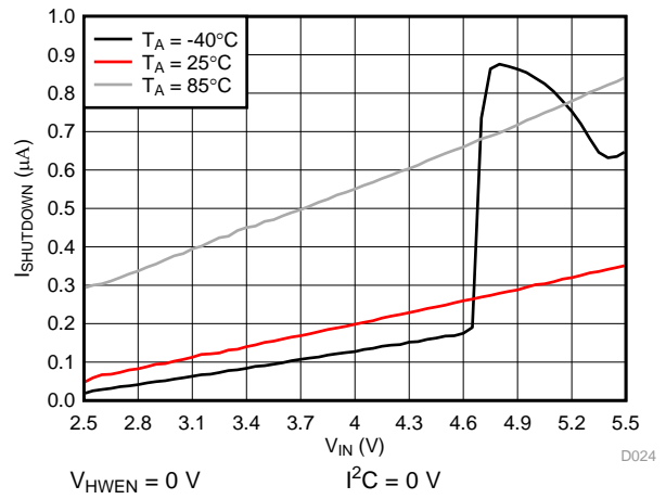
图 27. I_q Shutdown
