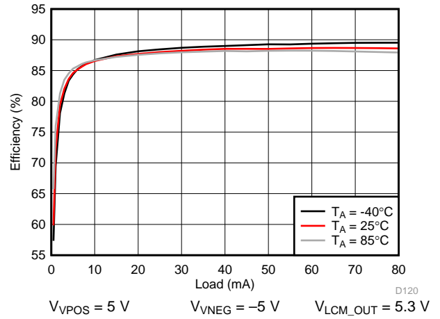
图 206. VPOS/VNEG Efficiency
