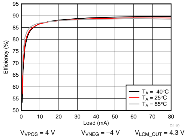
图 205. VPOS/VNEG Efficiency
