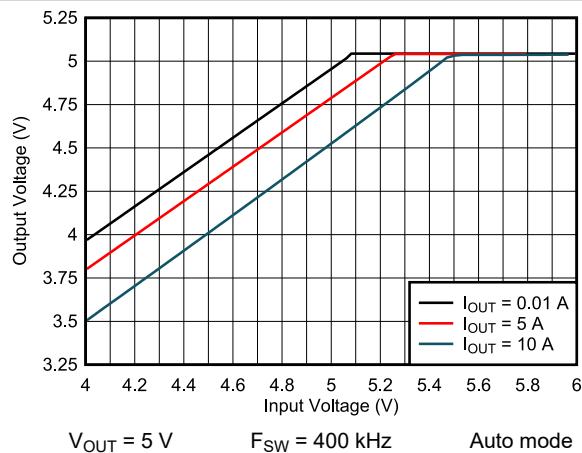
图 9-21. Dropout
