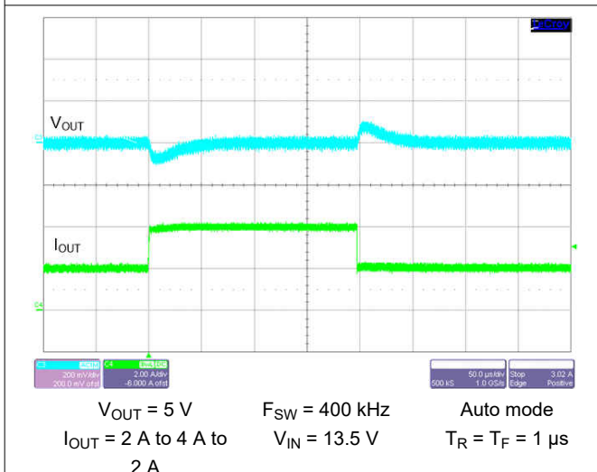
图 9-39. Load Transient
