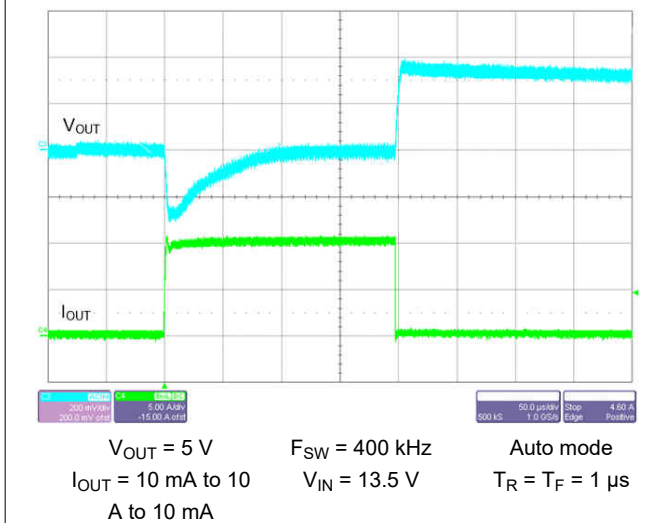
图 9-37. Load Transient
