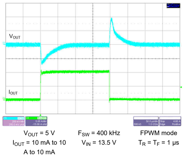
图 9-38. Load Transient
