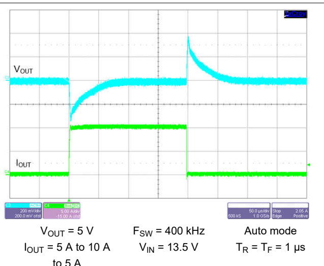
图 9-40. Load Transient
