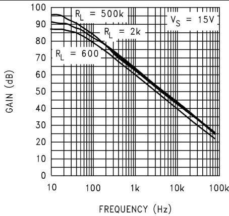
图 21. 开环频率响应
