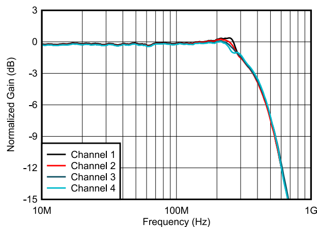
闭环带宽
