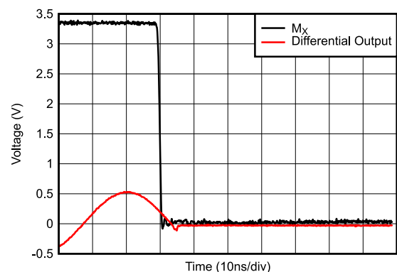
图 6-16. Turn-Off Time
