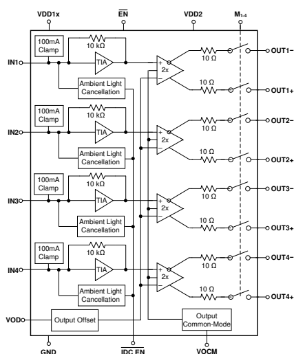
简化版方框图
