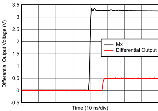
图 6-15. Turn-On Time
