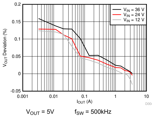
图 5-5. 负载调整率
