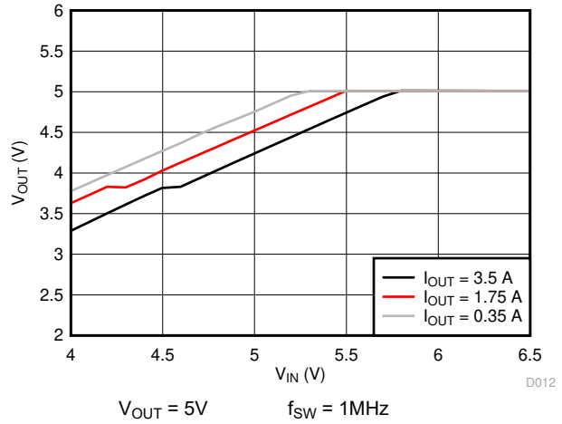
图 5-8. 压降曲线
