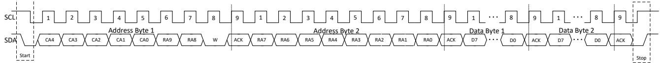
图 8-11. I 2 C Write Timing
