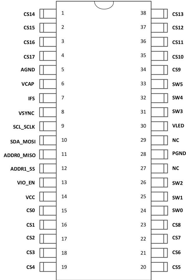
图 6-2. LP5866 VQFN Package 38-Pin VQFN Top View
