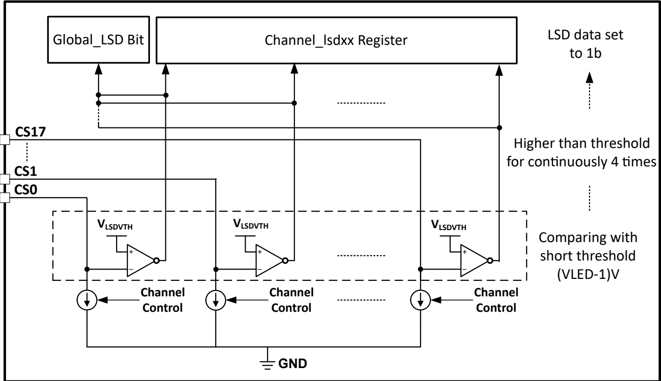
图 8-12. LSD Circuit
