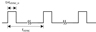
图 8-10. VSYNC Timing
