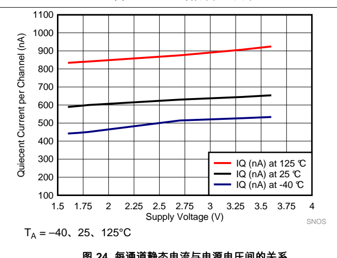
图 24. 每通道静态电流与电源电压间的关系
