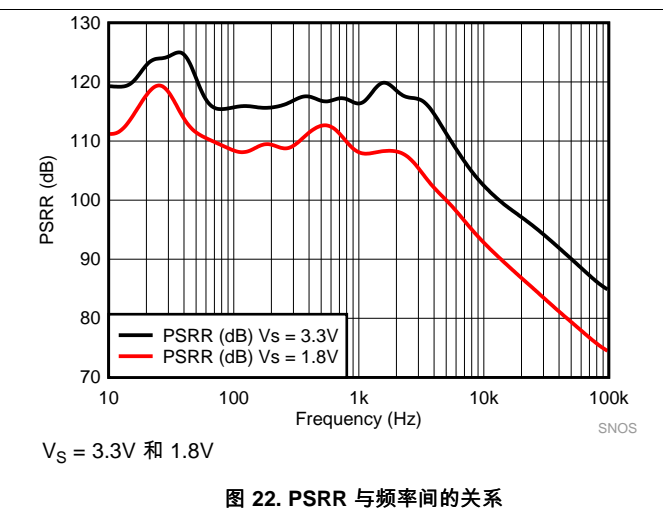
图 22. PSRR 与频率间的关系
