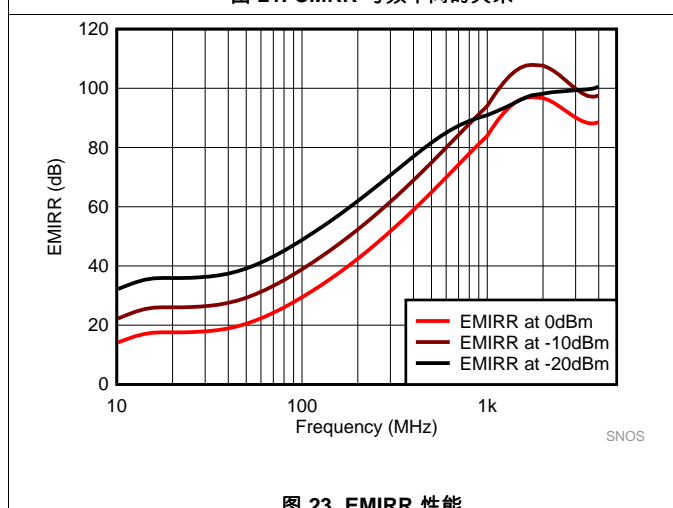
图 23. EMIRR 性能
