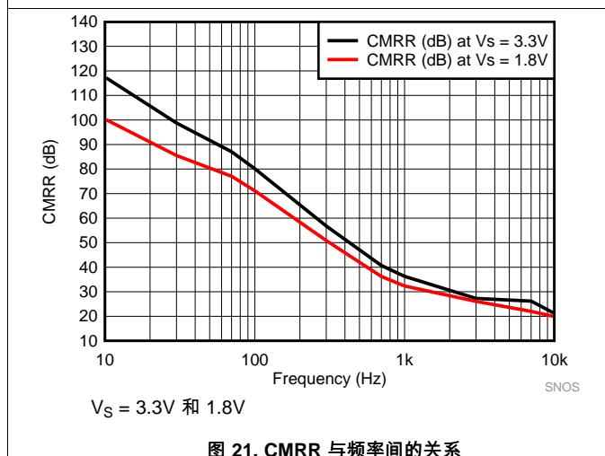
图 21. CMRR 与频率间的关系
