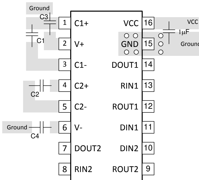
图 7-3. MAX232E Layout
