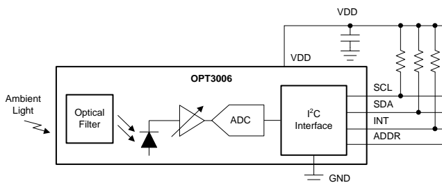
方框图
