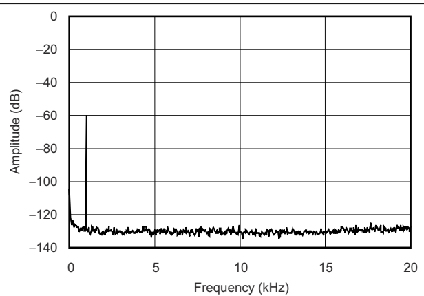
图 6-10. Output Spectrum
