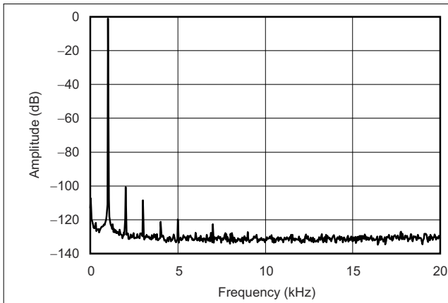
图 6-9. Output Spectrum
