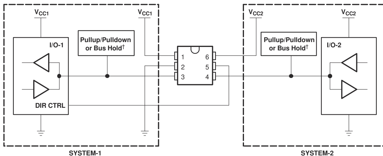
图 8-3. 双向逻辑电平转换应用
