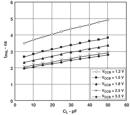
图 5-4. 低电平到高电平的典型传播延迟与负载电容间的关系 T A = 25°C、V CCA = 1.5V
