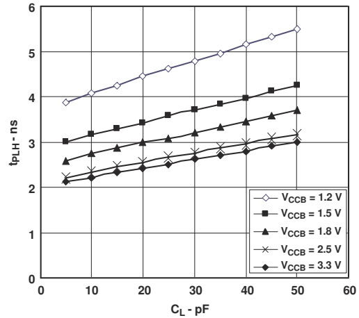
图 5-2. 低电平到高电平的典型传播延迟与负载电容间的关系 T A = 25°C、V CCA = 1.2V
