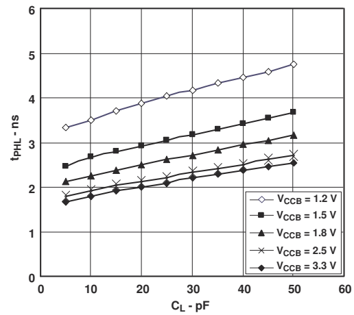
图 5-6. 低电平到高电平的典型传播延迟与负载电容间的关系 T A = 25°C、V CCA = 1.8V
