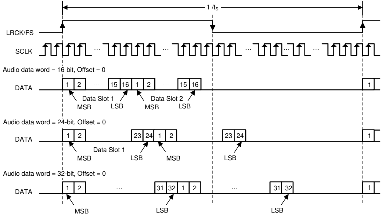
图 8-5. TDM 1 Audio Data Format
