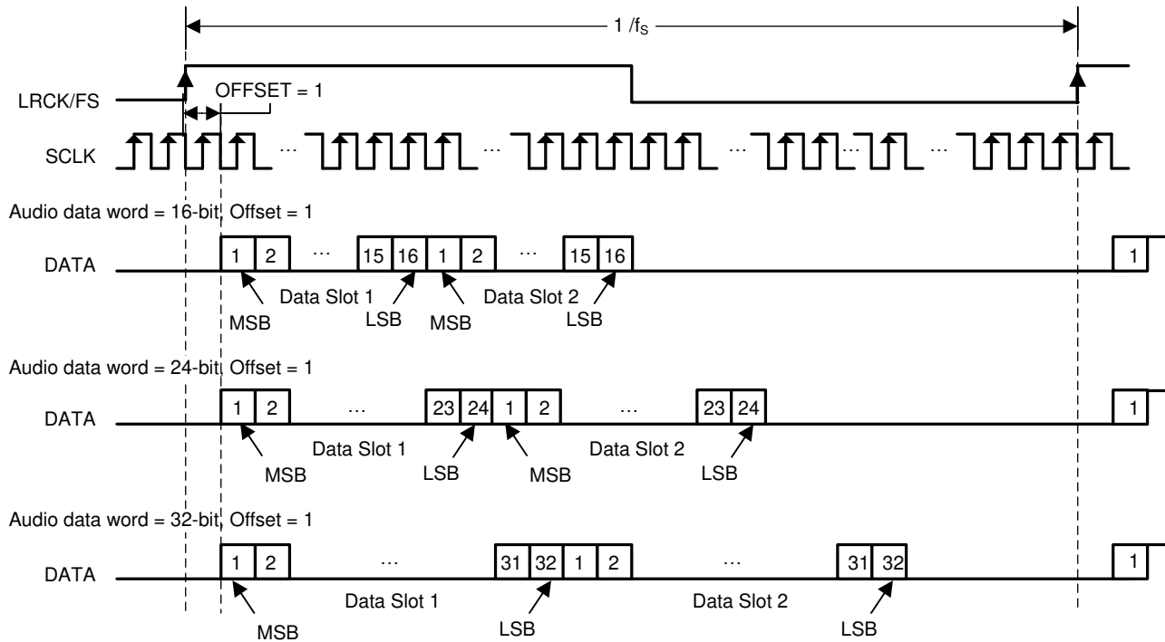
图 8-5. TDM 1 Audio Data Format
