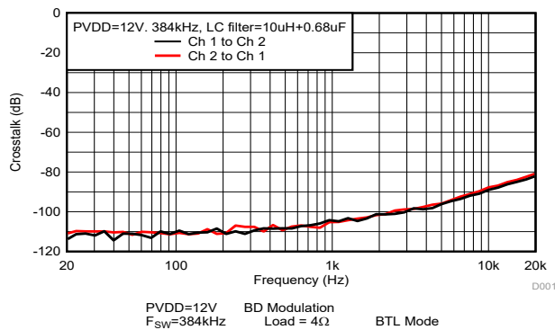
图 6-15. Crosstalk
