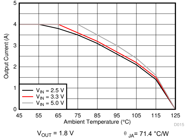
图 8-15. Thermal Derating
