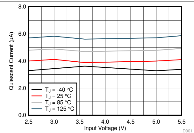
图 6-4. Quiescent Current
