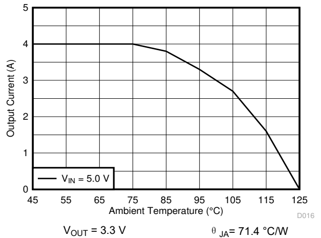
图 8-17. Thermal Derating
