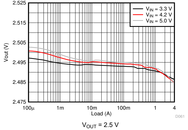
图 8-9. Load Regulation
