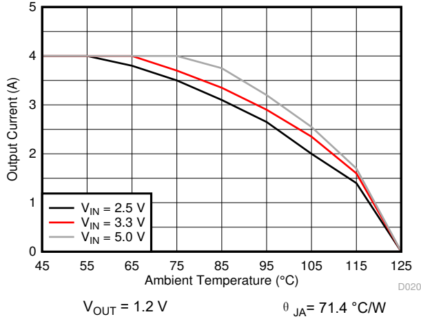
图 8-14. Thermal Derating
