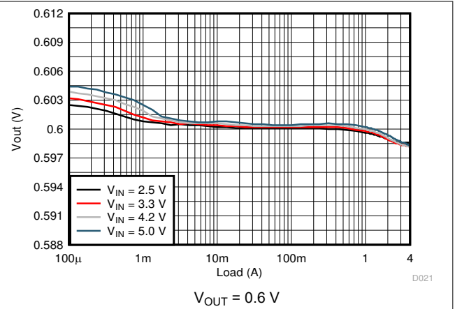
图 8-3. Load Regulation
