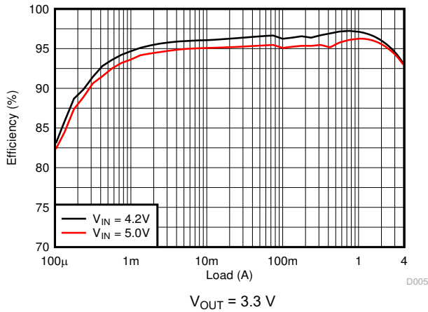
图 8-10. Efficiency
