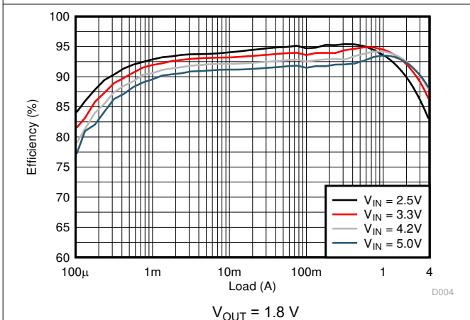
图 8-6. Efficiency
