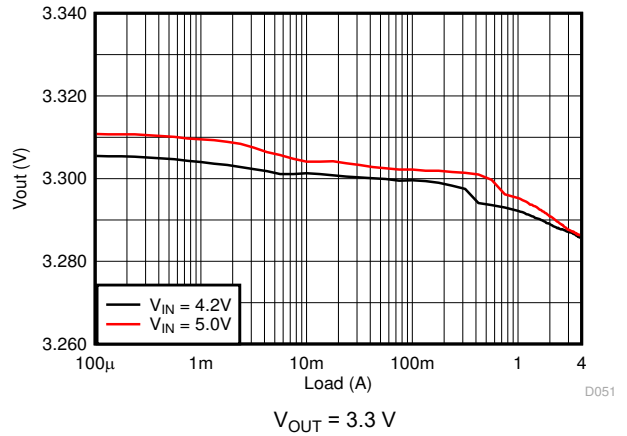
图 8-11. Load Regulation
