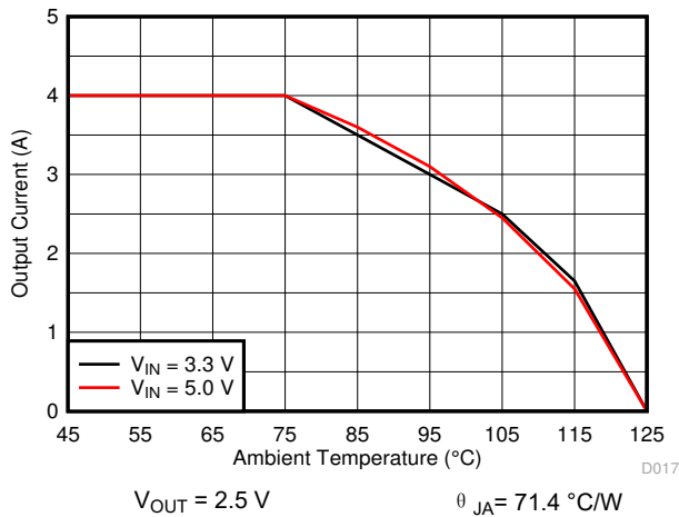
图 8-16. Thermal Derating
