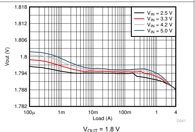
图 8-7. Load Regulation
