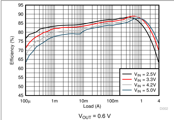
图 8-2. Efficiency
