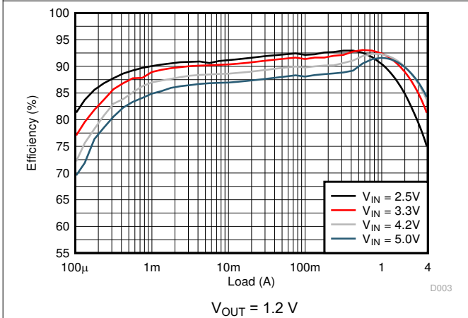
图 8-4. Efficiency
