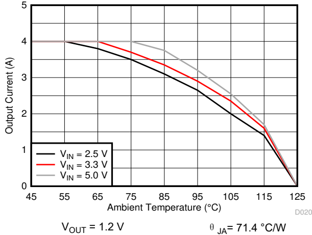
图 8-14. Thermal Derating
