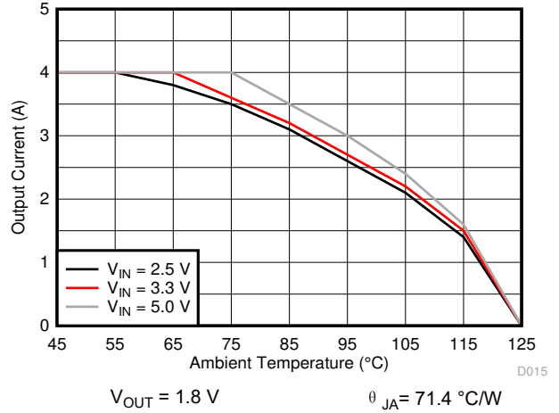
图 8-15. Thermal Derating
