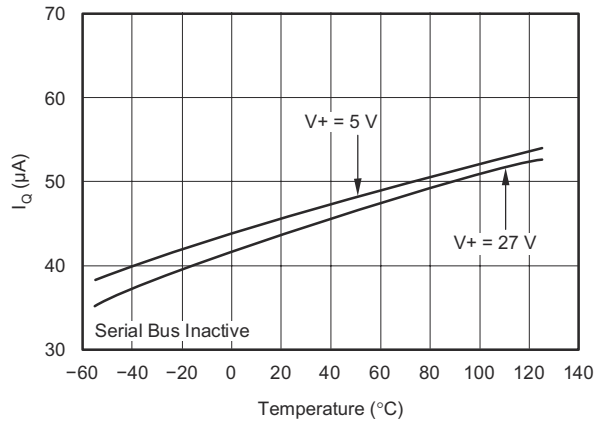
图 6-1. 静态电流与温度间的关系
