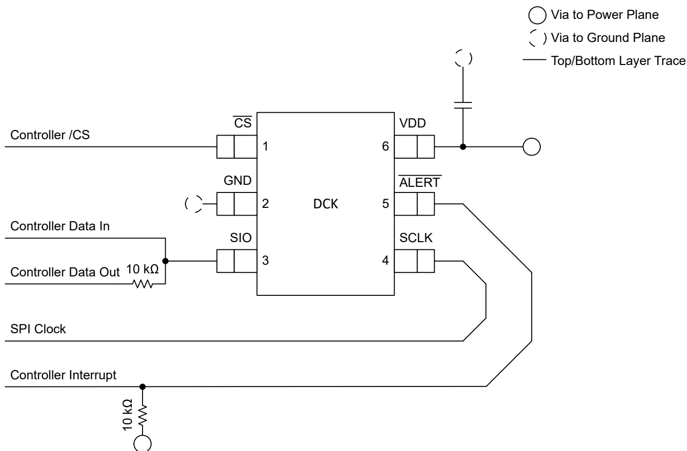
图 11-1. DCK 封装布局示例
