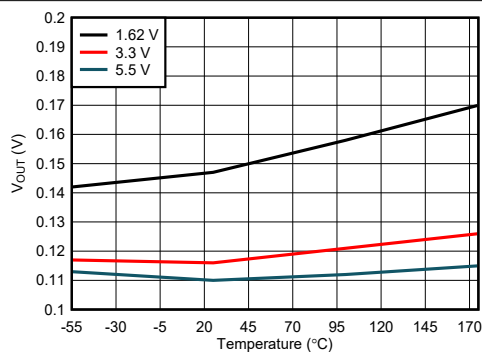
图 7-9. ALERT 输出与温度间的关系
