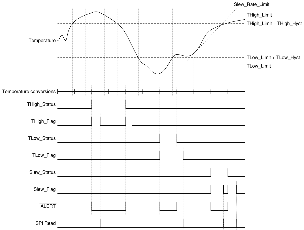
图 8-8. 比较器模式时序图
