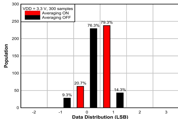
图 7-4. -55°C 时的温度测量噪声分布
