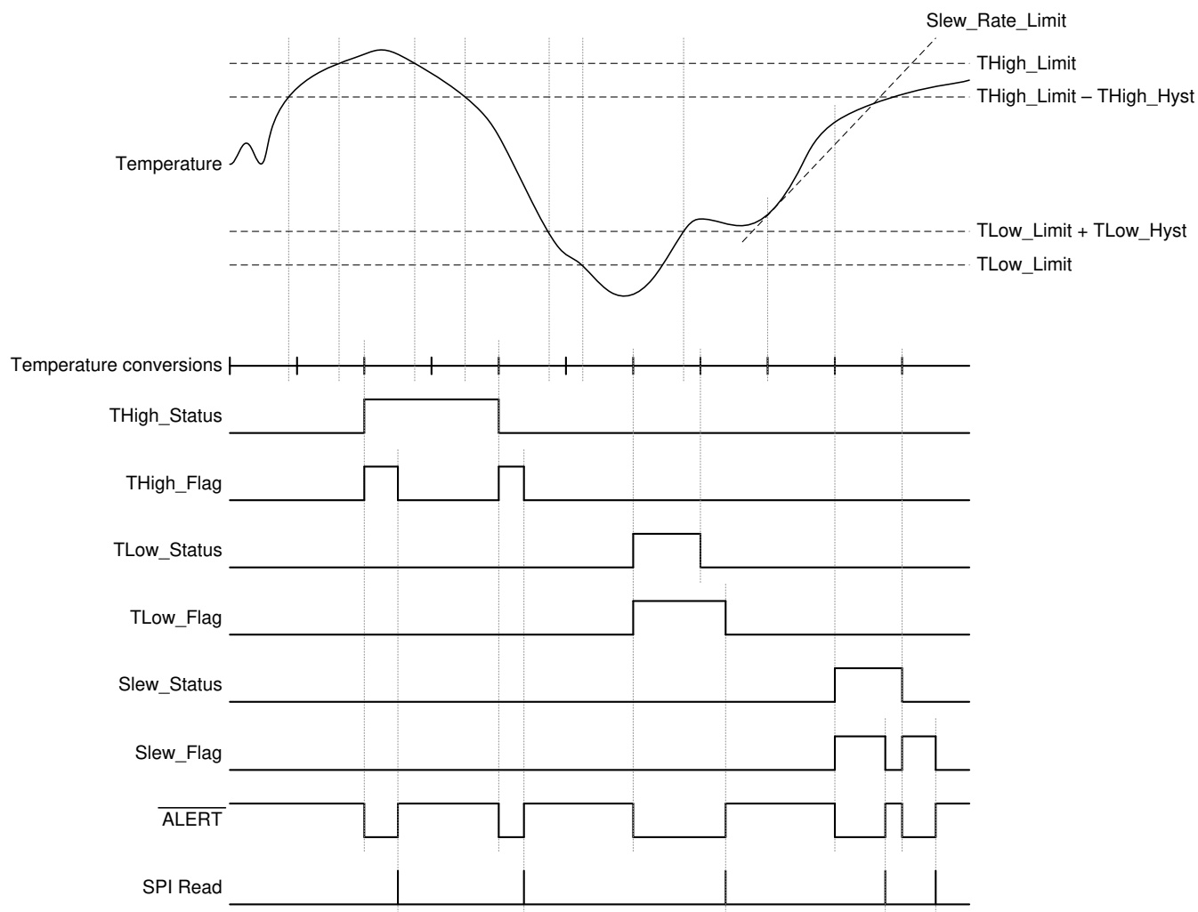
图 8-7. 中断模式图
