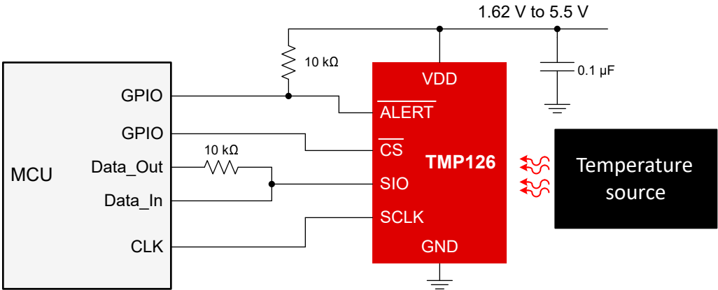
图 9-1. TMP126 典型连接
