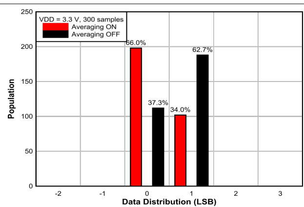
图 7-3. 25°C 时的温度测量噪声分布
