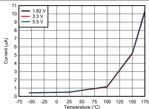
图 7-7. 待机电流与温度间的关系
