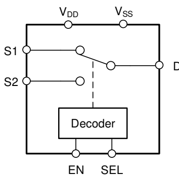
方框图
