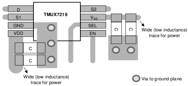
图 11-2. TMUX7219DQK Layout Example
