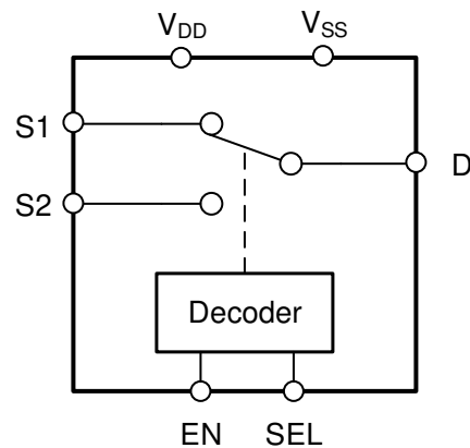
功能方框图
