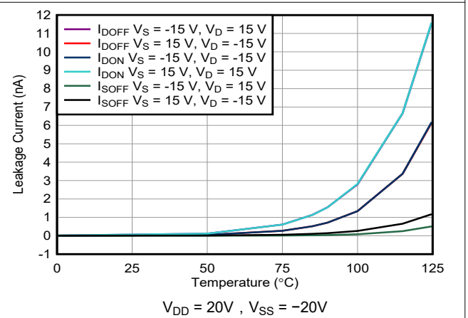
图 7-16. 泄漏电流与温度间的关系
