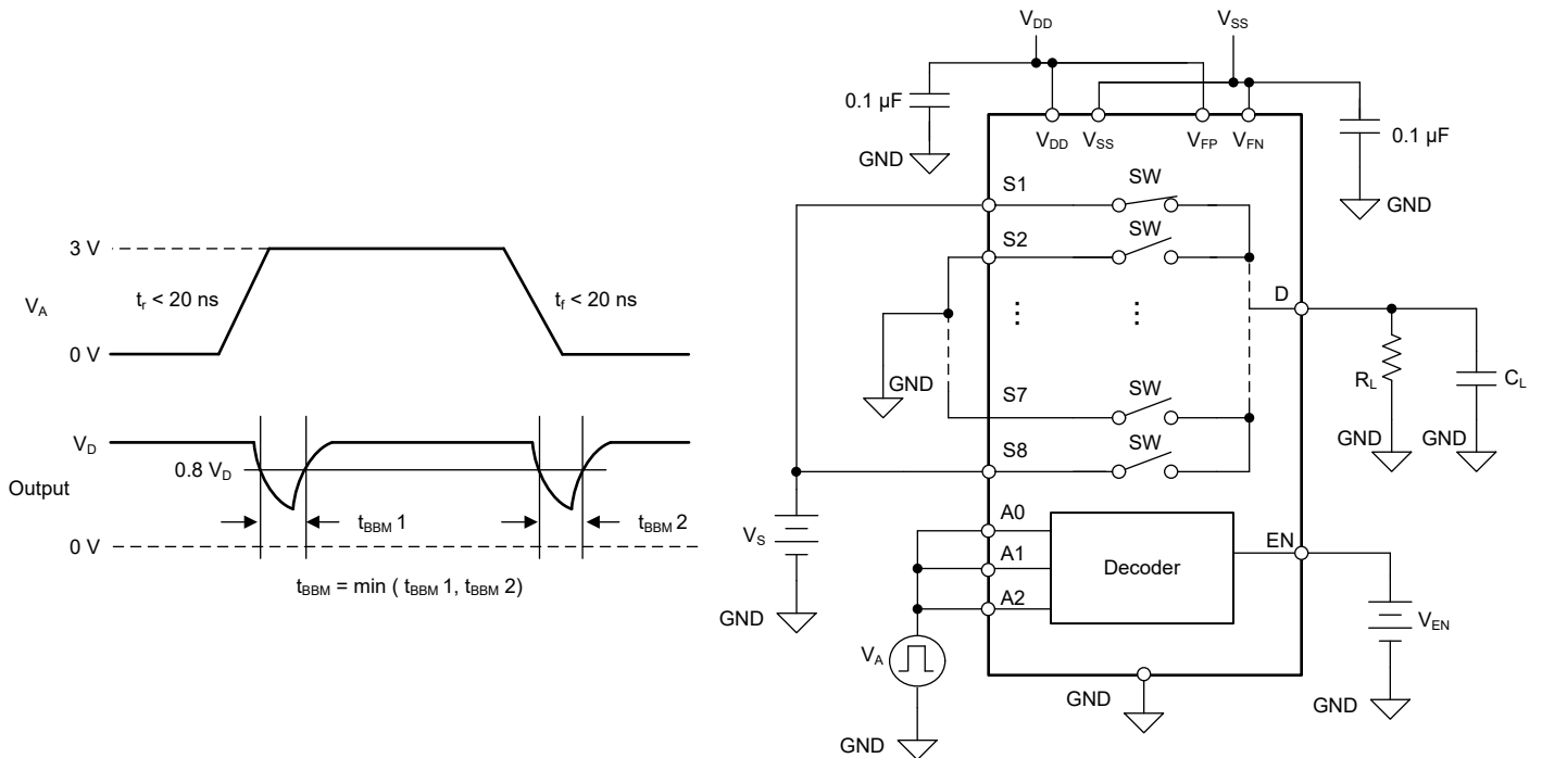
图 8-6. 先断后合延迟测量设置
