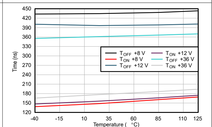
图 7-28. 转换时间与温度间的关系
