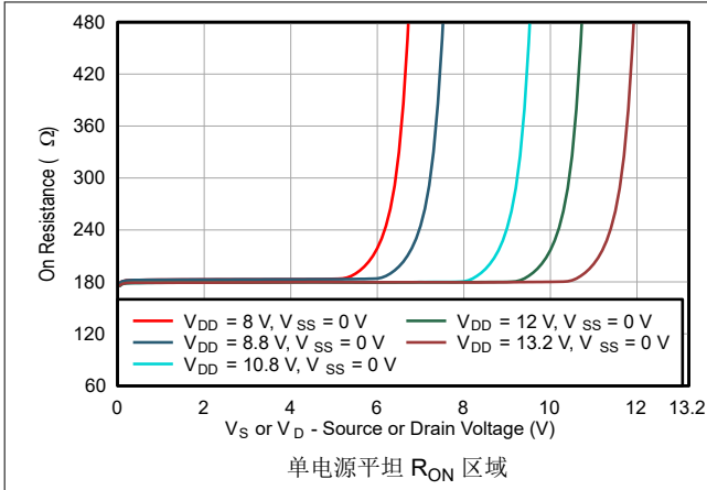
图 7-7. 导通电阻与源极或漏极电压之间的关系
