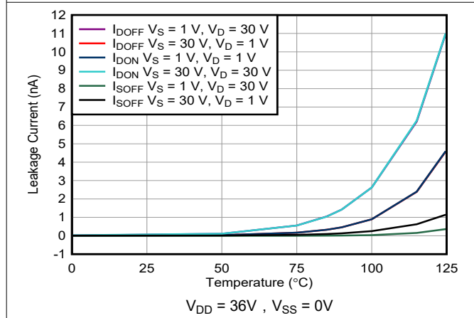
图 7-15. 泄漏电流与温度间的关系
