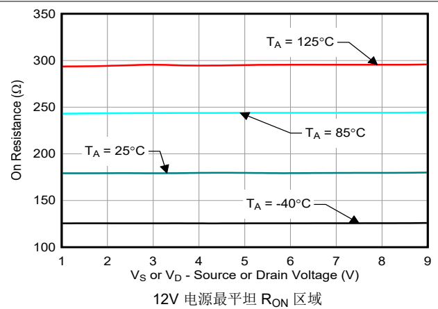
图 7-8. 导通电阻与源极或漏极电压之间的关系
