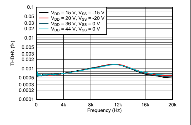
图 7-24. THD+N 与频率间的关系
