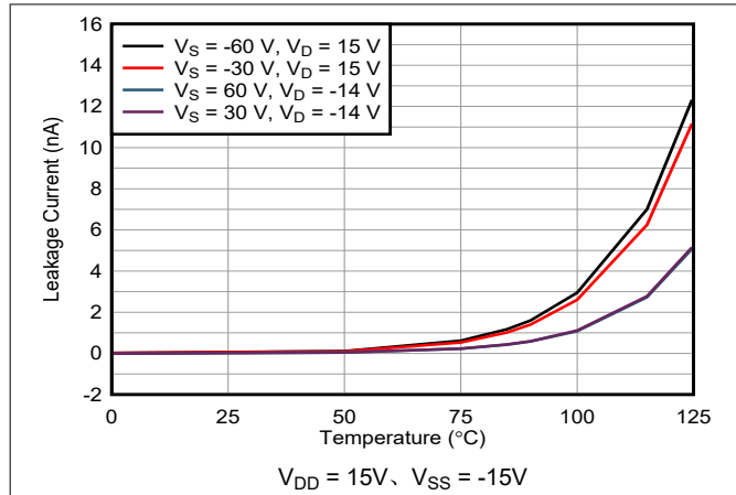
图 7-19. I_{D(FA)} 过压漏电流与温度的关系
