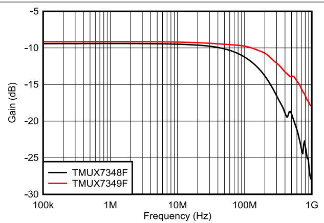
图 7-32. 导通响应与频率间的关系
