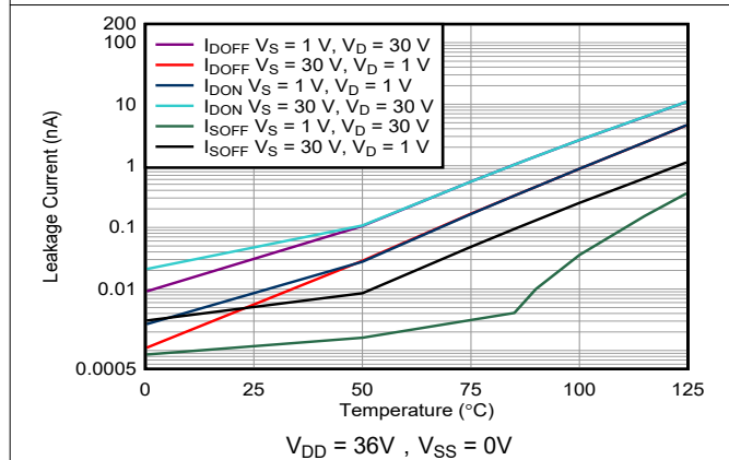
图 7-17. 泄漏电流与温度间的关系
