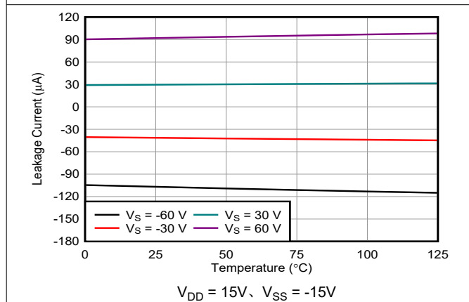
图 7-23. I_{S(FA)} 过压漏电流与温度的关系
