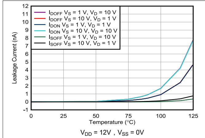
图 7-13. 泄漏电流与温度间的关系
