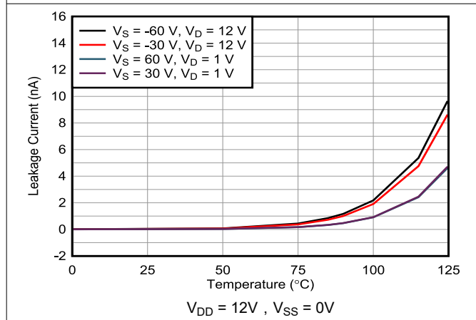
图 7-21. I_{D(FA)} 过压漏电流与温度的关系
