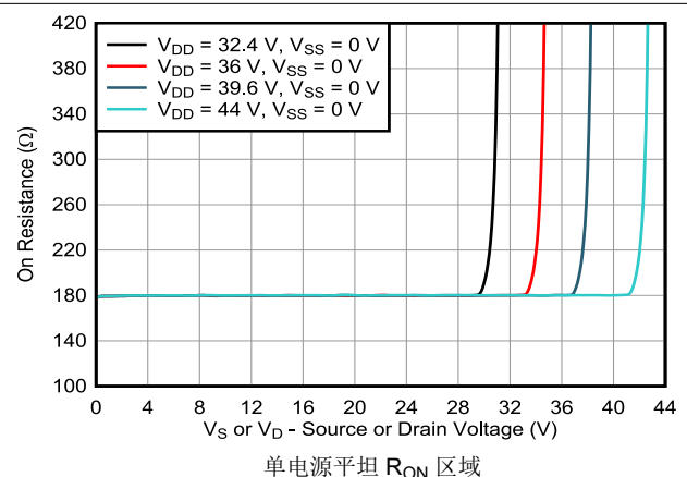
图 7-10. 导通电阻与源极或漏极电压之间的关系
