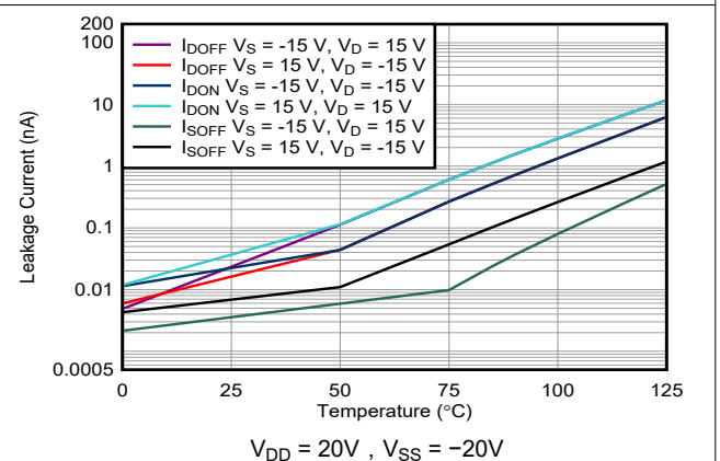
图 7-18. 泄漏电流与温度间的关系
