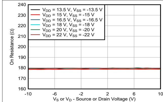
图 7-3. 导通电阻与源极或漏极电压之间的关系
