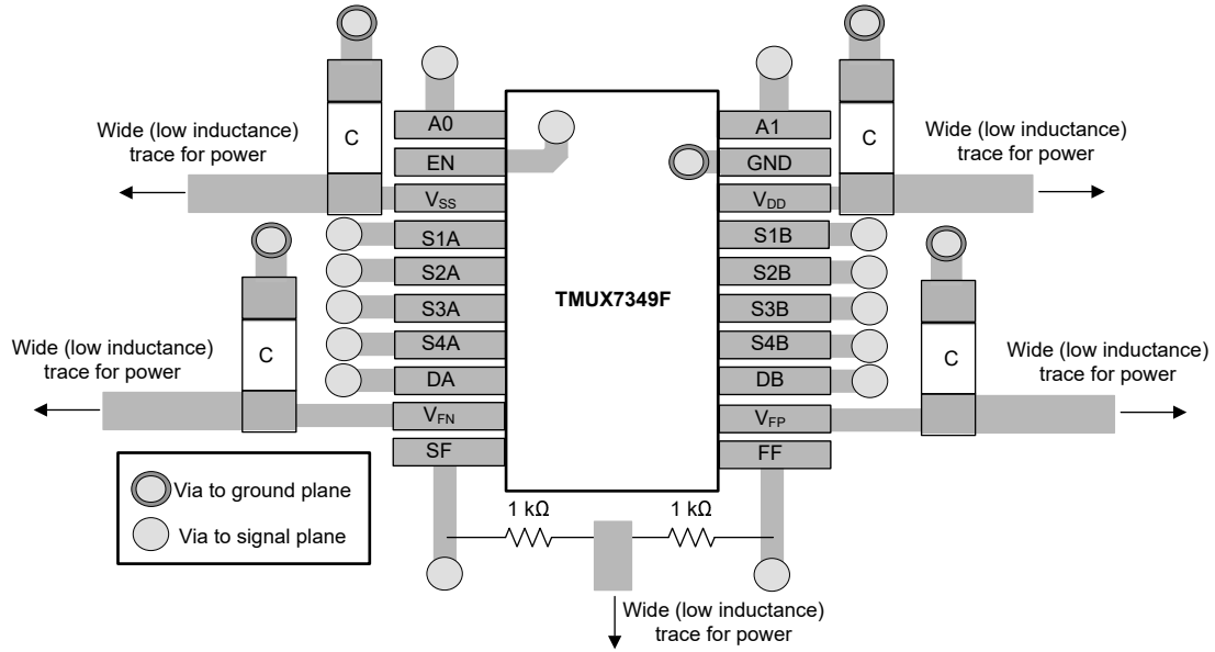
图 10-5. TMUX7349FPW 布局示例
