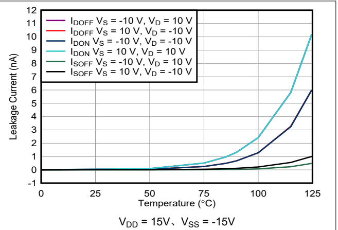
图 7-14. 泄漏电流与温度间的关系
