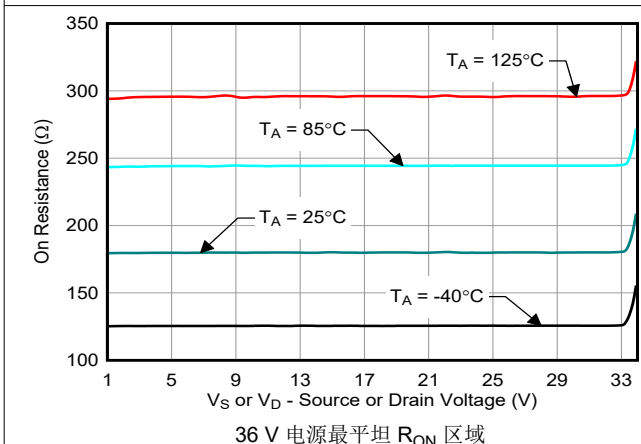
图 7-11. 导通电阻与源极或漏极电压之间的关系
