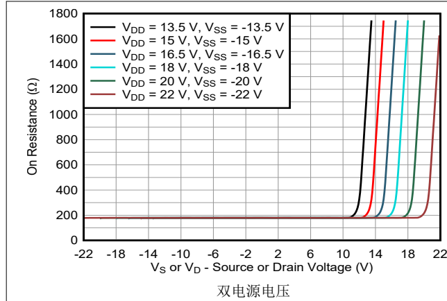
图 7-1. 导通电阻与源极或漏极电压之间的关系
