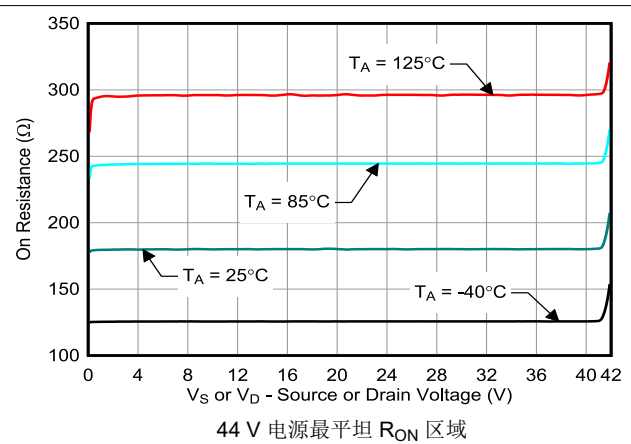
图 7-12. 导通电阻与源极或漏极电压之间的关系
