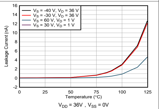
图 7-22. I_{D(FA)} 过压漏电流与温度的关系
