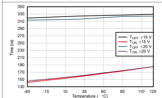
图 7-27. 转换时间与温度间的关系
