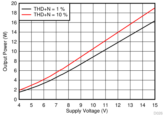
A. Load = 4 Ω , 1SPW
