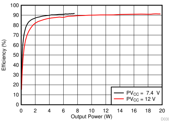
A. Load = 8 Ω , 1SPW
