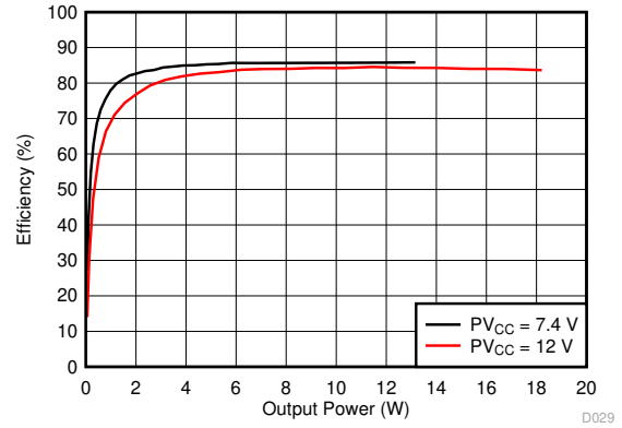
A. Load = 4 Ω , 1SPW
