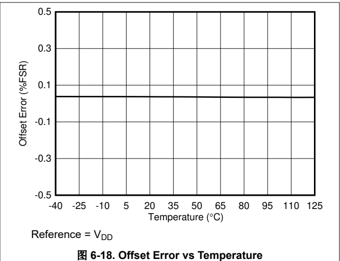
图 6-18. Offset Error vs Temperature
