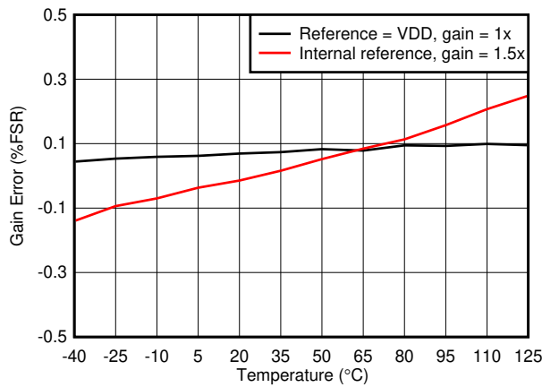
图 6-9. Gain Error vs Temperature
