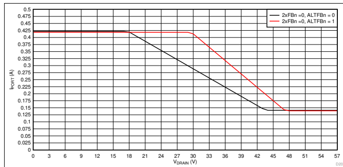
图 92. 1x 模式 (2xFBn = 0) 折返曲线， I_{PORT} 与 V_{DRAIN} 间的关系
