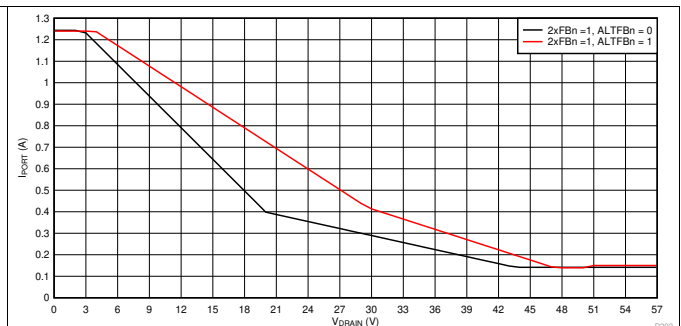
图 93. 2x 模式 (2xFBn = 1) 折返曲线， I_{PORT} 与 V_{DRAIN} 间的关系
