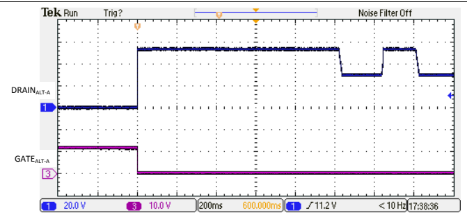
图 121. 由于 PCut 故障导致的 2 线对退避
