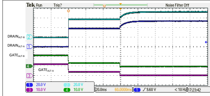
图 122. 4 线对 I_{LIM} 折返和关闭
