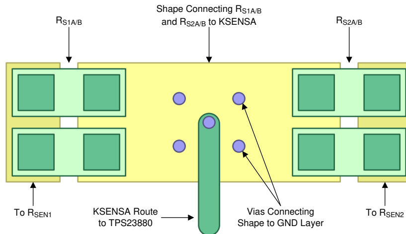
图 145. 开尔文检测布局示例
