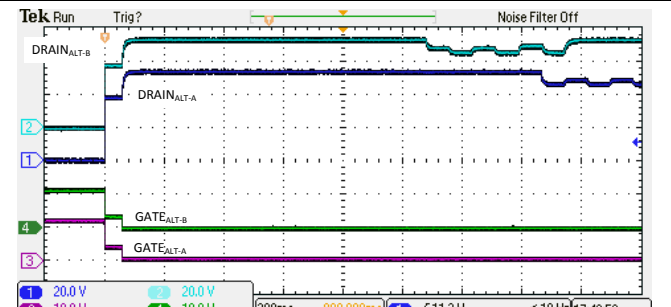
图 123. 由于 I_{LIM} 故障导致的 4 线对退避
