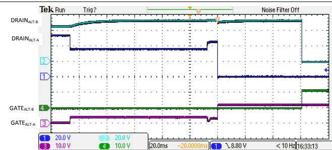
图 135. 4 线对单一特征 1 指分级和开启
