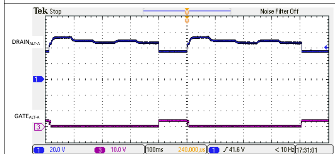
图 130. 具有有效 0-3 级负载的 2 线对半自动模式发现
