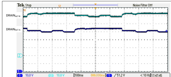
图 128. 4 线对低电阻 (11kΩ) 检测特征
