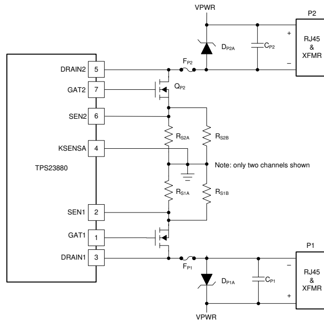
图 144. 开尔文电流检测连接
