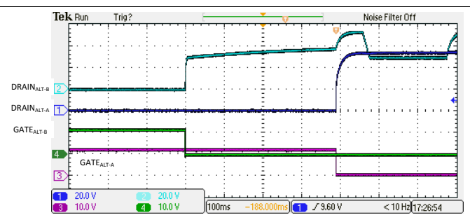
图 125. 4 线对单一特征 0-4 级断开
