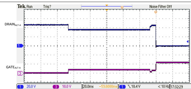
图 131. 2 线对 1 指分级和开启
