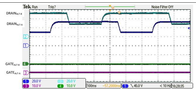
图 127. 4 线对开路检测特征
