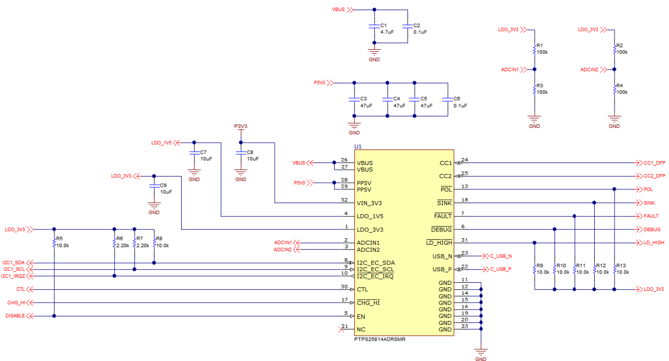
图 11-1. Example Schematic
