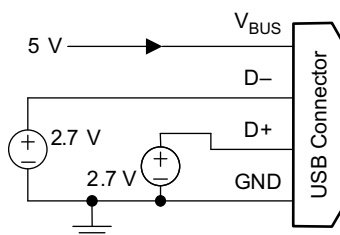
图 10-16. Divider 3 Mode
