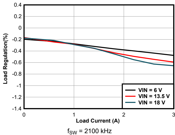
图 11-6. Load Regulation
