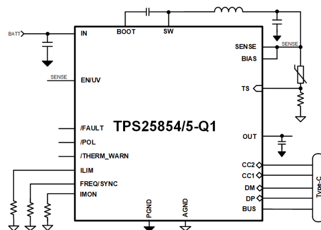
简化版原理图：TPS25845-Q1 和 TPS25855-Q1
