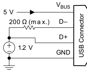
图 10-13. 1.2-V Mode
