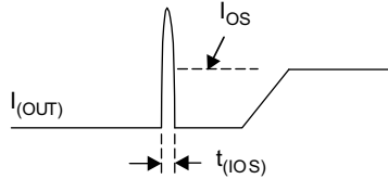
图 9-5. Output Short-Circuit Parameters
