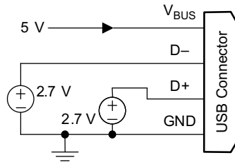
图 10-12. Divider 3 Mode
