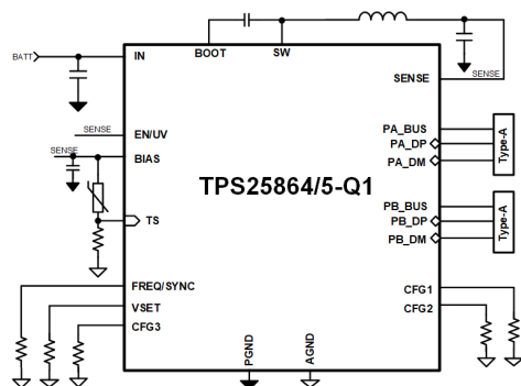
简化版原理图 TPS25864-Q1、TPS25865-Q1
