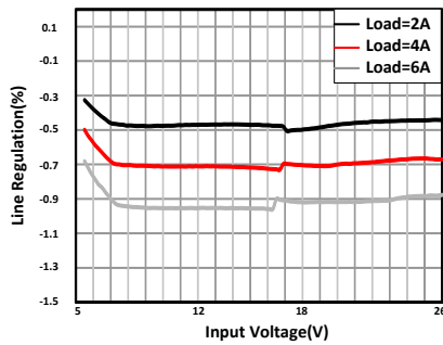
图 11-6. Line Regulation
