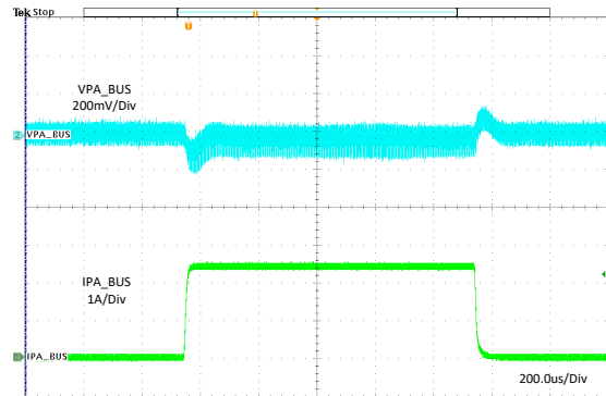
图 11-5. Load Regulation
