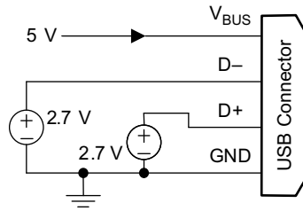
图 10-12. Divider 3 Mode
