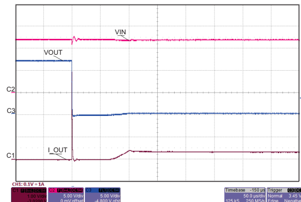
瞬态: 输出短路
