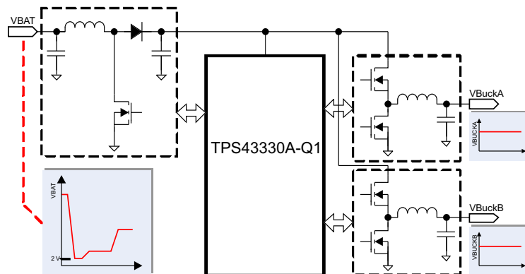
图 1. 典型应用图
