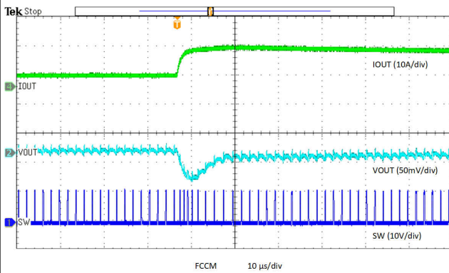
图 6-11. Load Transient
