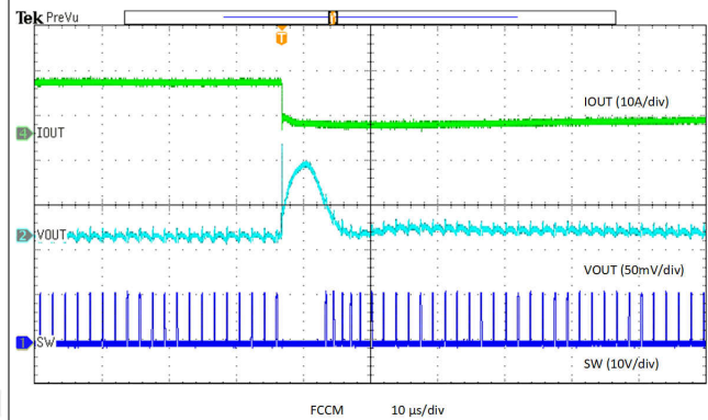
图 6-12. Unload Transient
