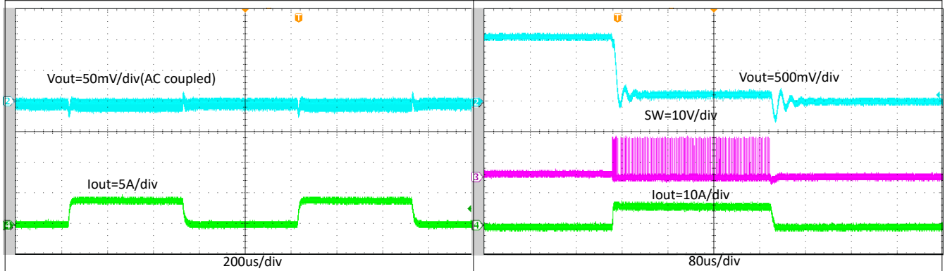
图 8-18. TPS564247 瞬态响应, 0.1A 至 4A, 负载阶跃为 2.5A/μs
