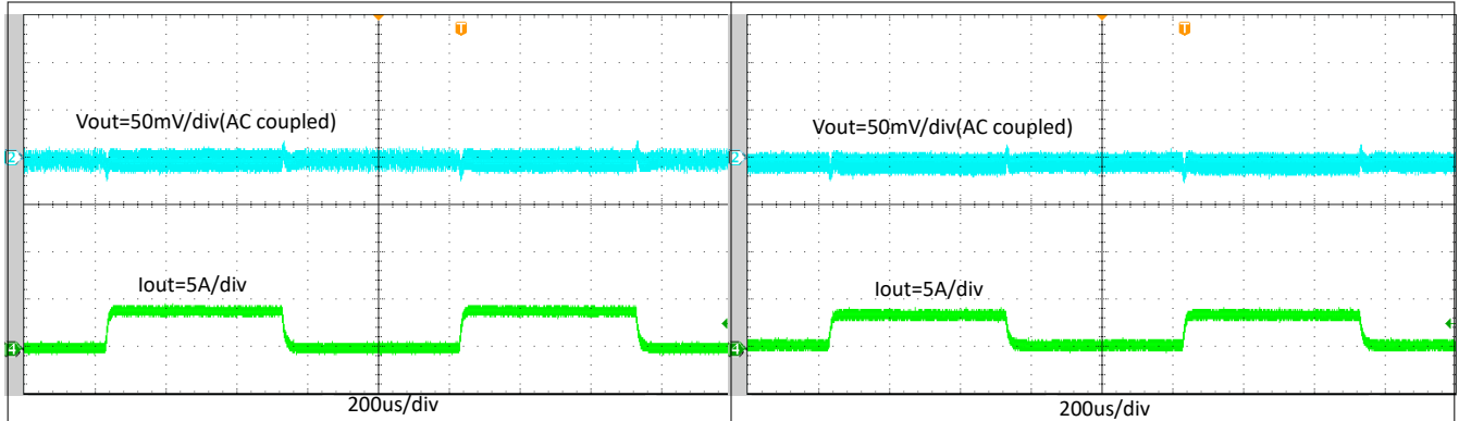
图 8-16. TPS564242 瞬态响应, 0.1A 至 4A, 负载阶跃为 2.5A/μs
