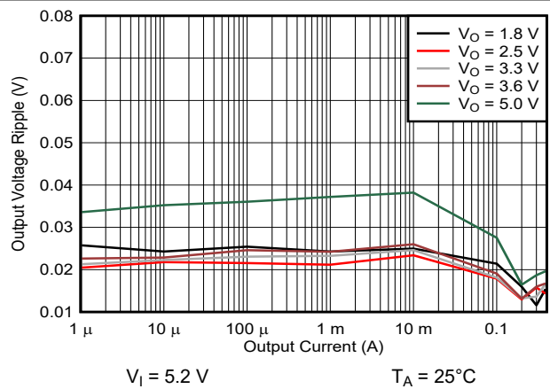
图 7-11. Output Voltage Ripple
