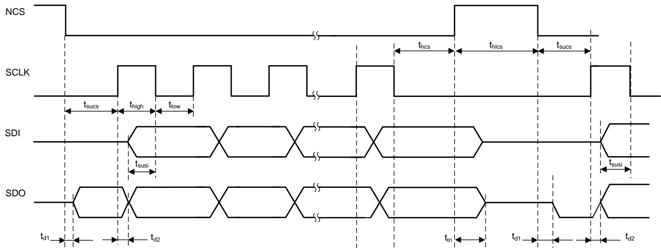
Figure 4-2. SPI 时序参数
