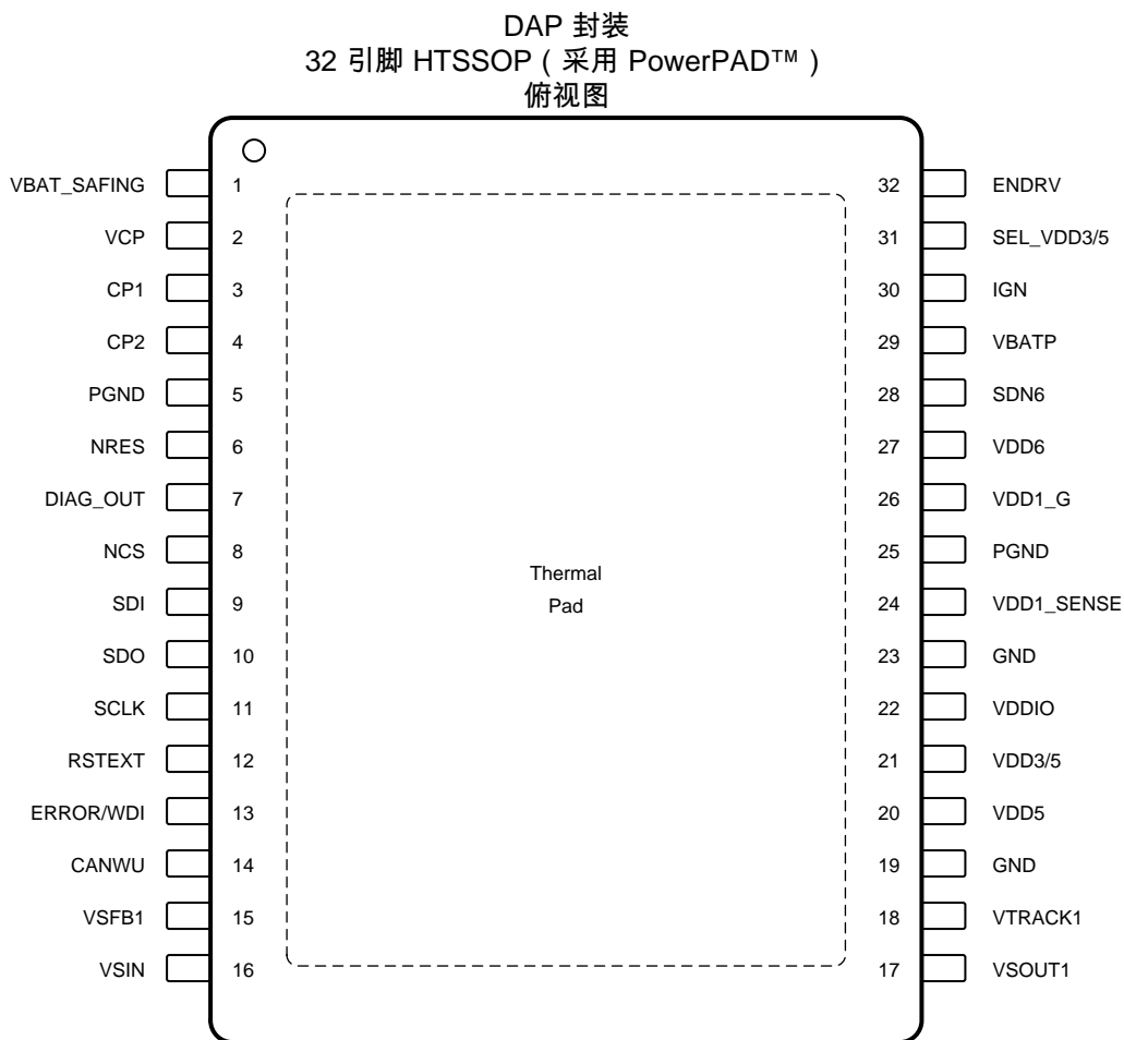
引脚功能
