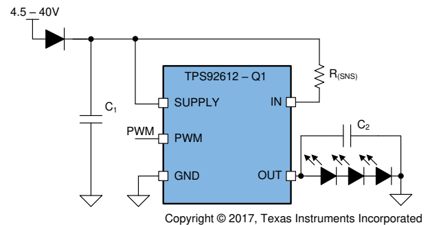
典型应用图
