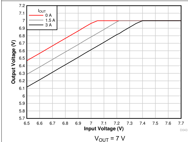
图 7-11. Voltage Dropout
