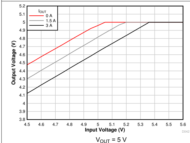
图 7-9. Voltage Dropout
