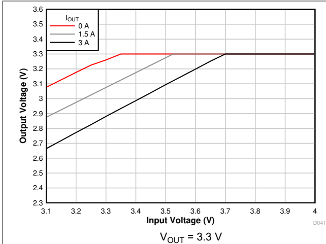
图 7-7. Voltage Dropout
