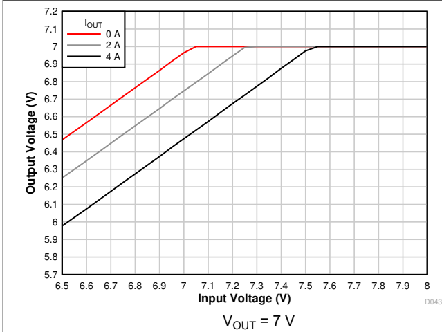
图 7-11. Voltage Dropout
