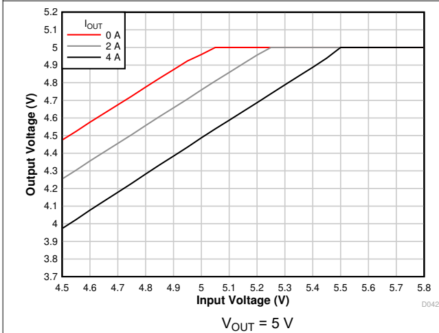
图 7-9. Voltage Dropout
