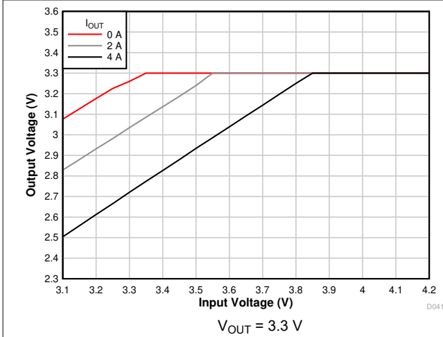
图 7-7. Voltage Dropout
