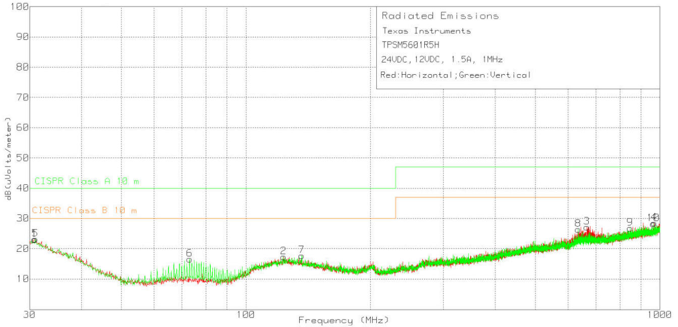
图 10-8. Radiated Emissions 24-V Input, 12-V Output, 1.5-A Load
