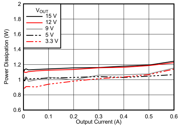
图 6-10. Power Dissipation
