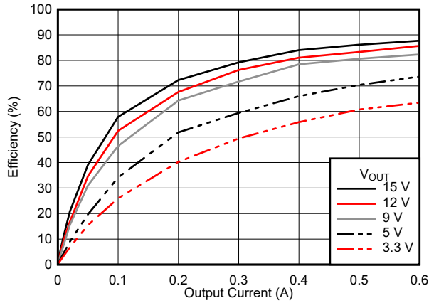
图 6-9. Efficiency
