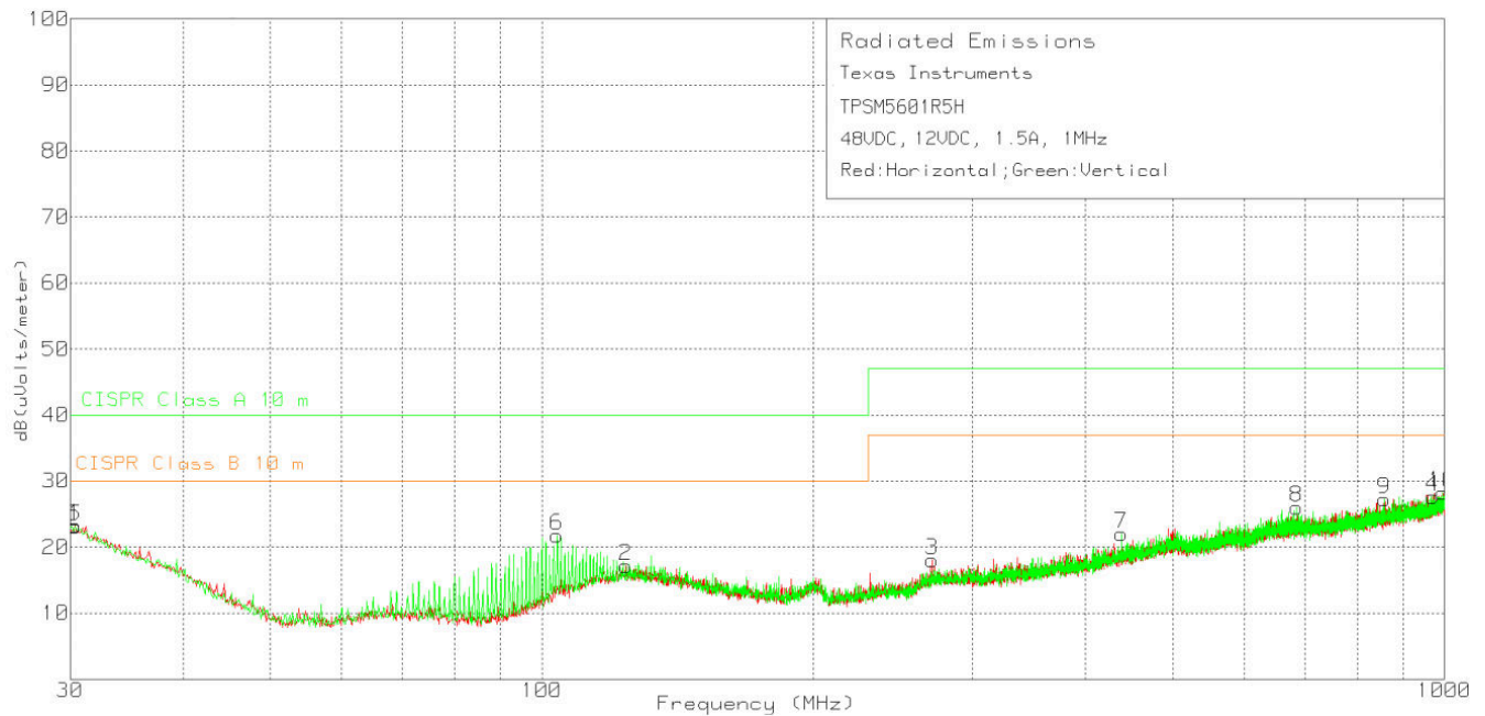
图 10-9. Radiated Emissions 48-V Input, 12-V Output, 1.5-A Load
