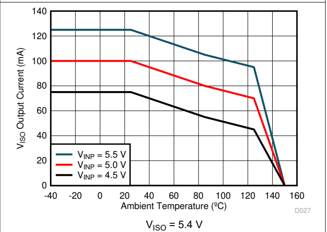
图 6-9. Maximum V_{ISO} Output Current vs. Temperature
