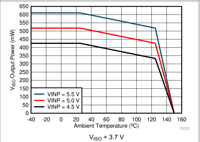
图 6-7. Maximum V_{ISO} Output Power vs. Temperature
