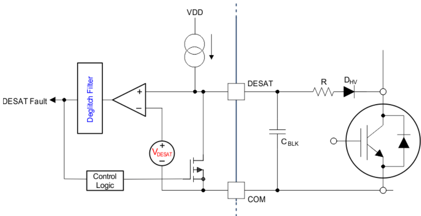
图 8-5. DESAT Protection
