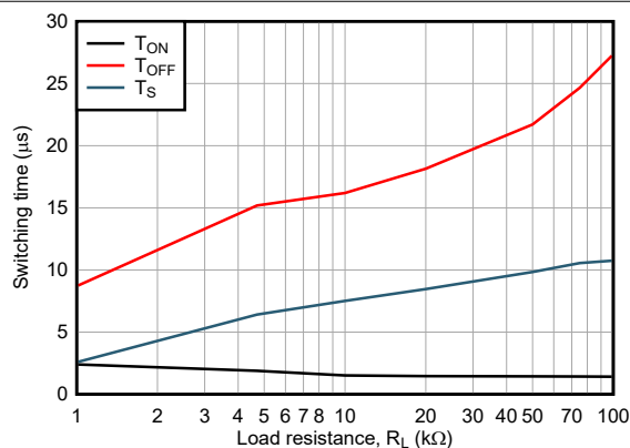
IF = 1.6mA ISOM8113-Q1 & ISOM8118-Q1 V CC = 5V
